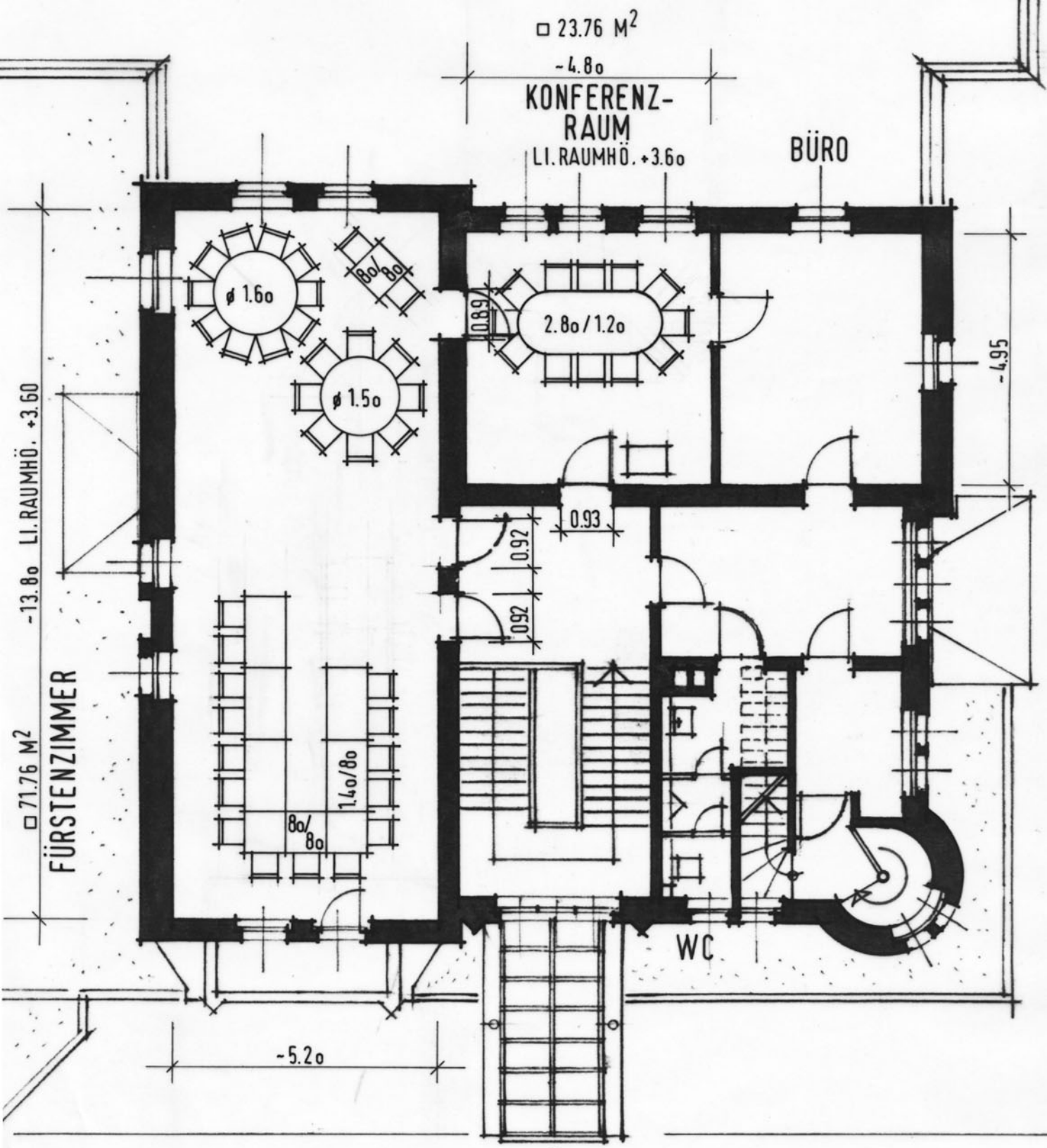
GRUNDRISS 1. OBERGESCHOSS BESTUHLUNGSVARIANTE
